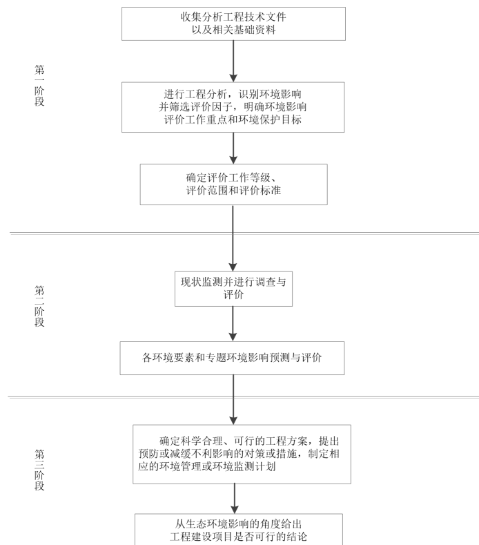
图 1.2-1 环境影响评价工作流程图
