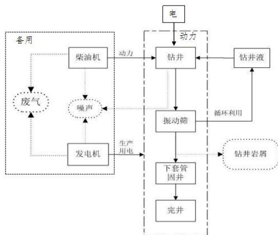
图 3.3-2 钻井工程施工过程及产污环节示意图
