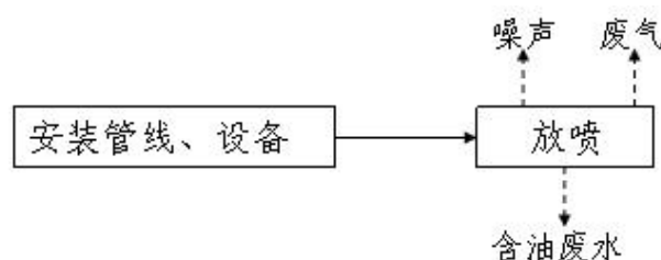
图 3.3-3 油气测试过程产污环节图
