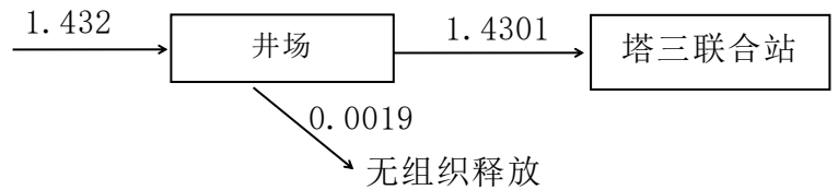
图 3.3-1 硫平衡图 单位：t/a
