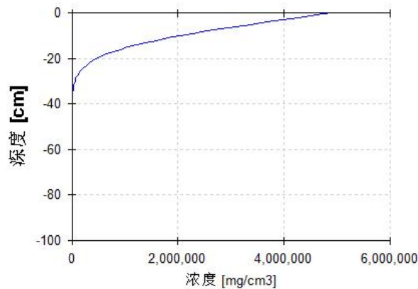
图 5.2-10 石油烃沿土壤垂向迁移情况
