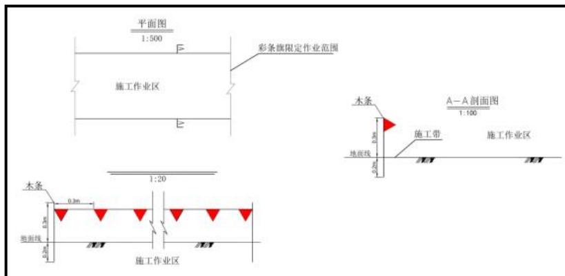
图 6.5-2 限行彩条旗典型措施设计图
