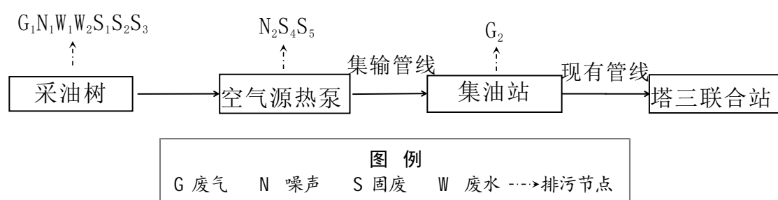
图 3.4-3 井场油气开采及集输工艺流程图
