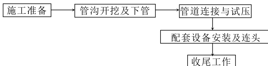
图3.4-2 施工方案工艺流程图
