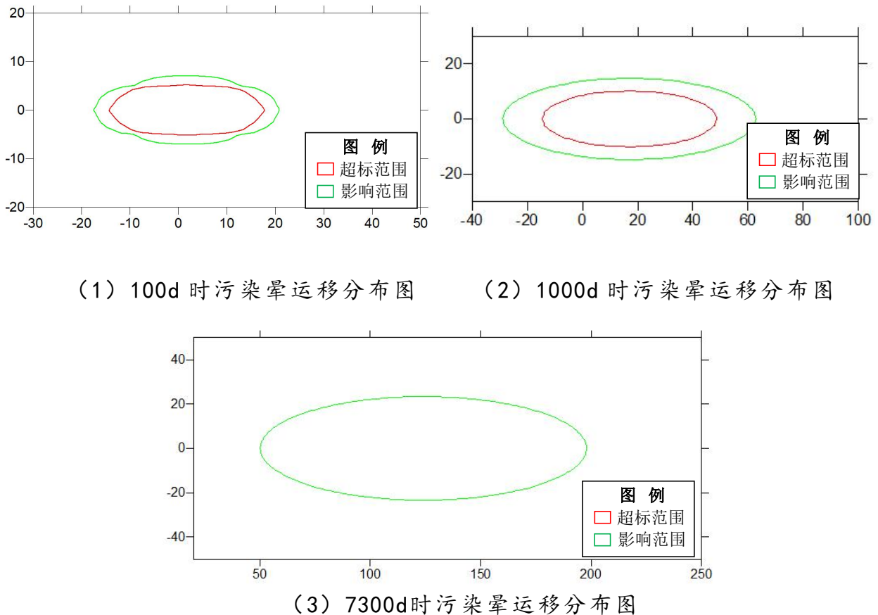
图 5.2-3 非正常状况下，石油类渗漏含水层影响范围图
