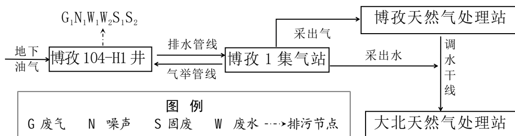
图图 3.4-9 气举排水井场集输和采出水输送工艺流程图
