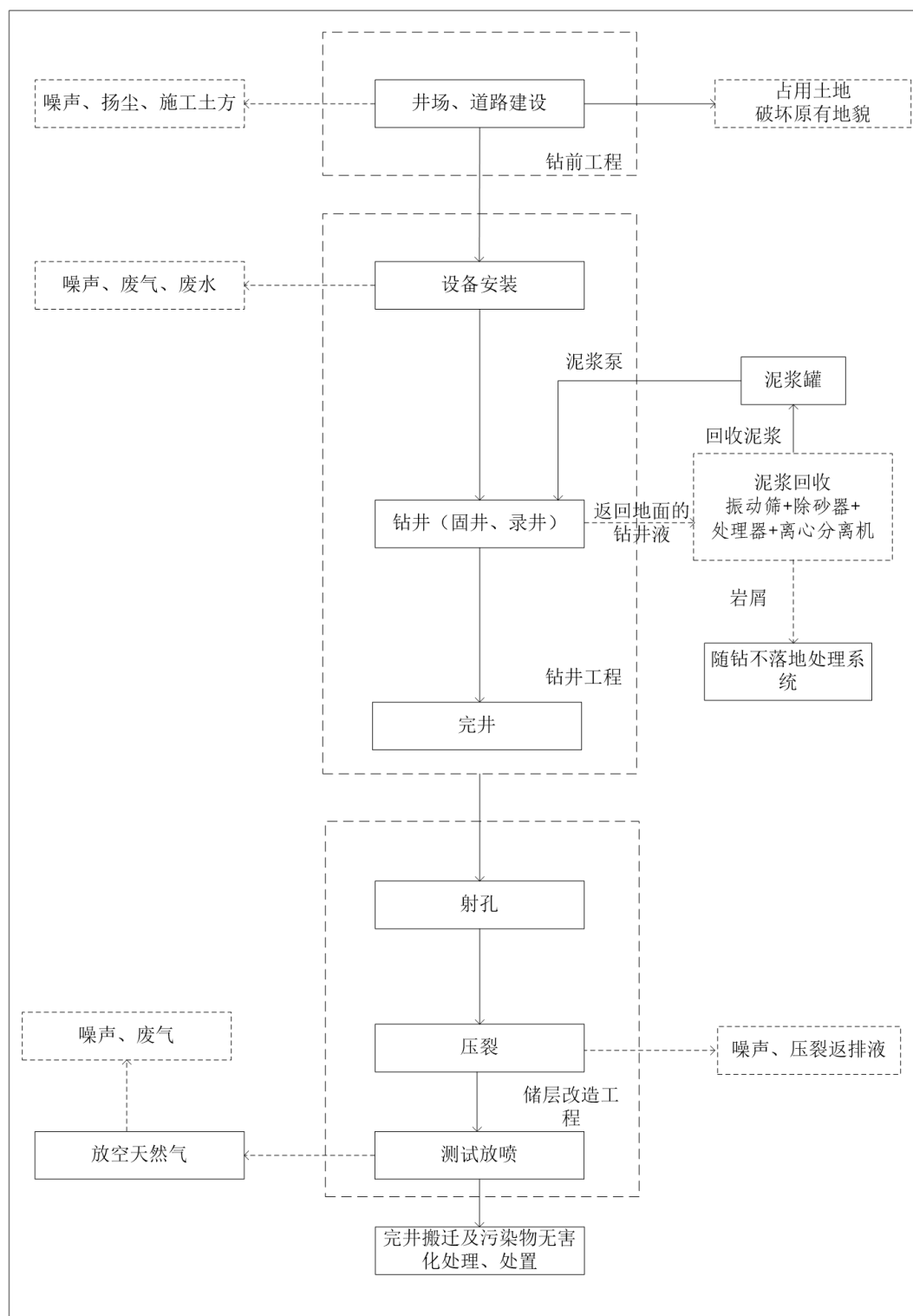
图 3.4-1 钻井工艺流程及污染物排放示意图
