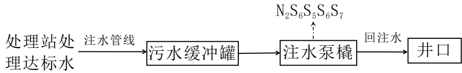
图图 3.4-10 大宛 3JS 井场注水工艺流程图
