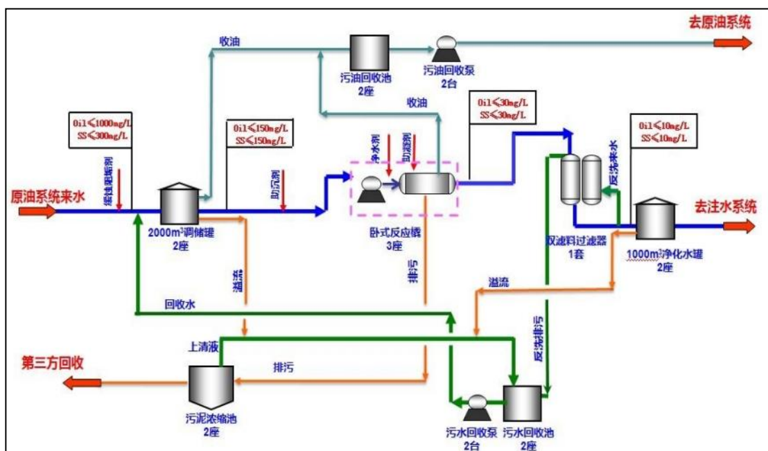
图 3.1-3 联合站水处理工艺流程图
