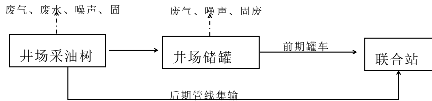
图 3.3-4 井场采油工艺流程图
