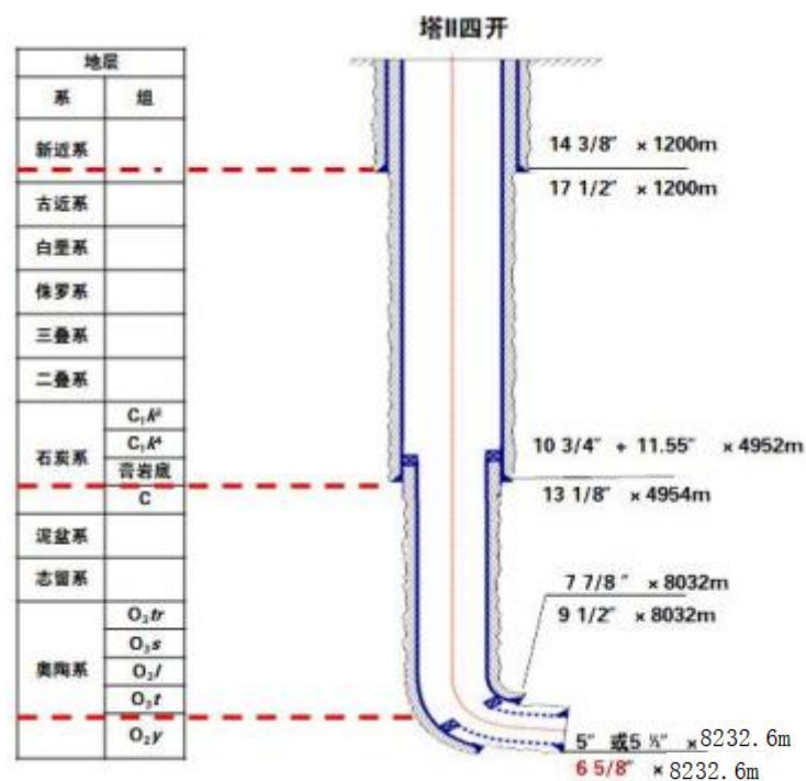
图2.3-1 井身结构示意图
