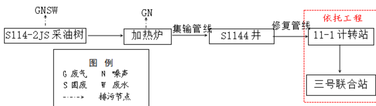
图 3.3-5 集输工艺流程图
