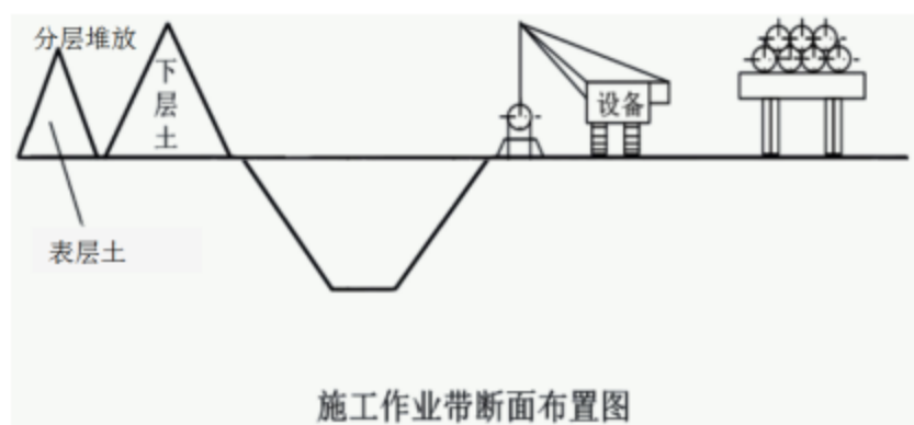
图 3.3-3 一般地段管道施工方式断面示意图
