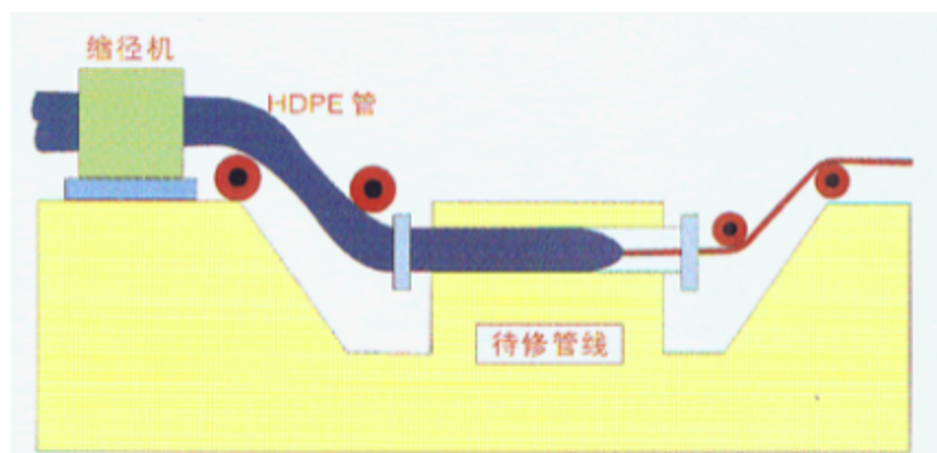
图3.3-5 管线内穿插修复施工作业示意图
