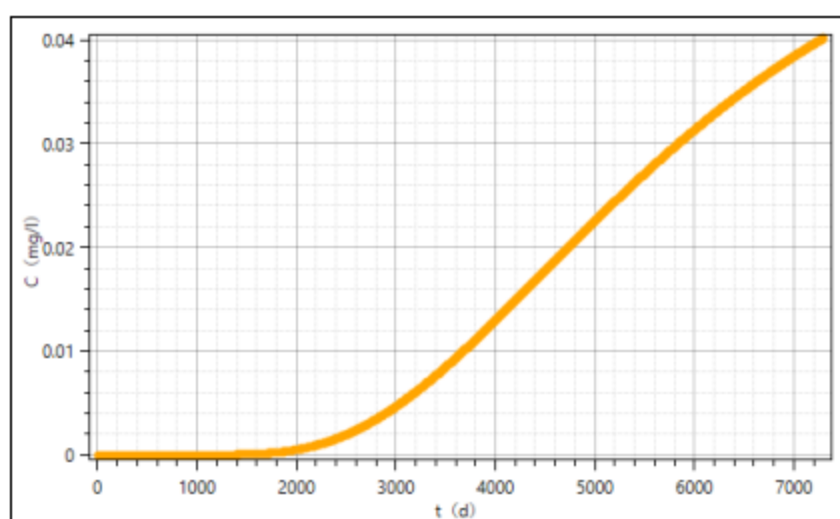
图5.2-3 井场非正常状况下，井场边界石油类浓度变化曲线图
