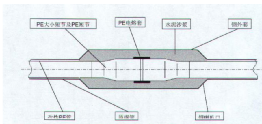
图3.3-6 内衬管连接示意图
