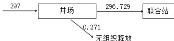
图 3.3-2 拟建工程井场硫平衡图 单位：kg/a
