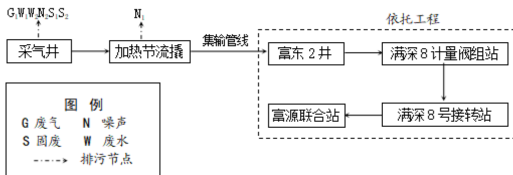
图 3.4-4 井场油气开采及集输工艺流程图
