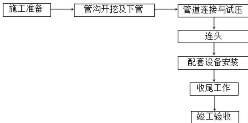
图 3.4-1 施工方案工艺流程图
