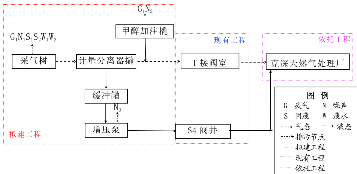
图 3.3-7 井场油气开采及集输工艺流程图
