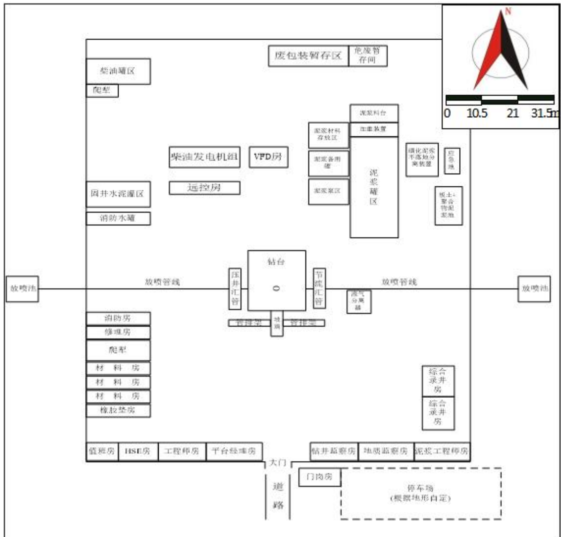
图 3 项目井场平面布置图
