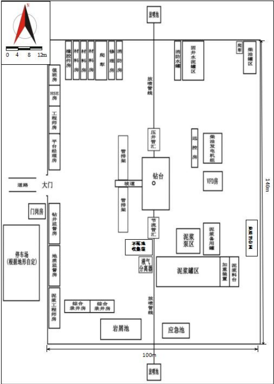
图 3.2-2 雄英 201 井场平面布置图
