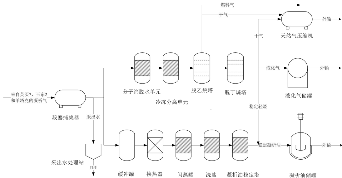
图 3.3-3 英买处理站油气处理流程图
