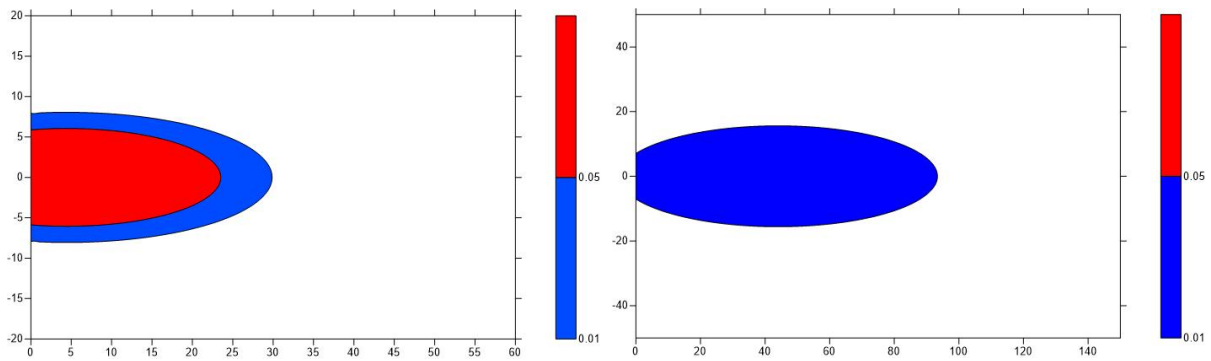
(1) 100d 时污染晕运移分布图
