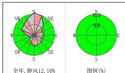
图 5.5-1 近 20 年风频玫瑰图
