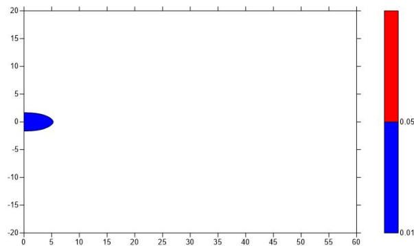
图 5.2-3 非正常状况下，石油类渗漏含水层影响范围图（10d）
