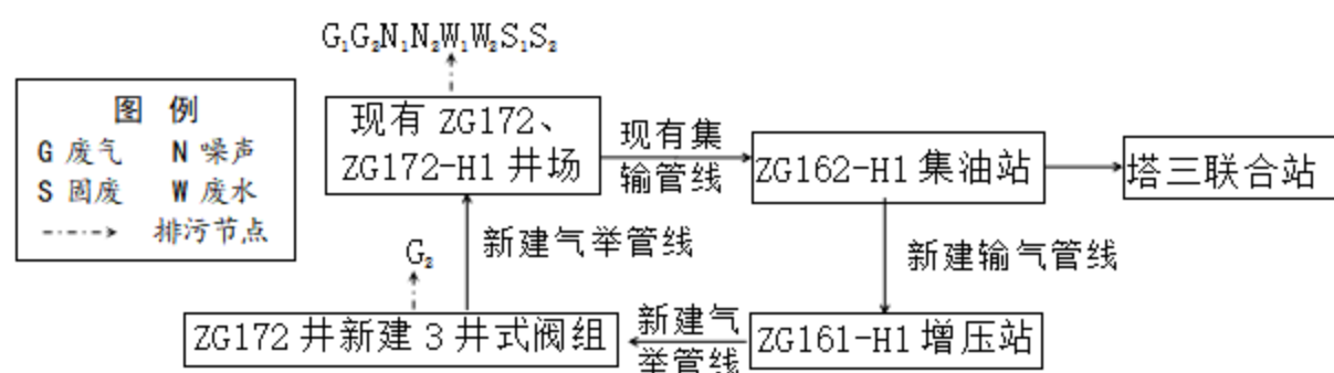
图 3.3-3 井场油气开采及集输工艺流程图
