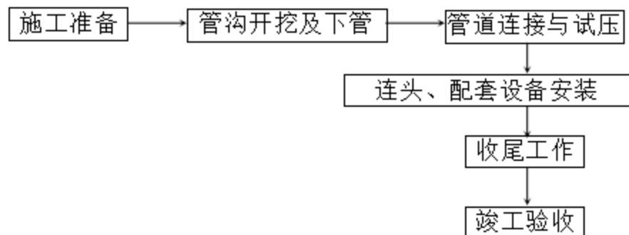
图3.3-2 施工方案工艺流程图
